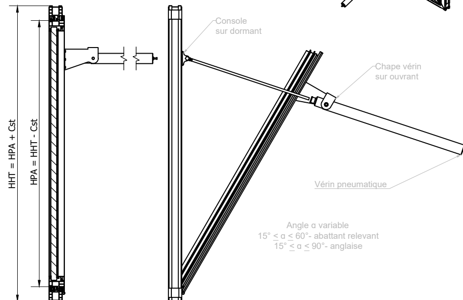
A-A ( 1:10 )
