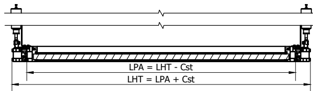
B-B ( 1:10 )
